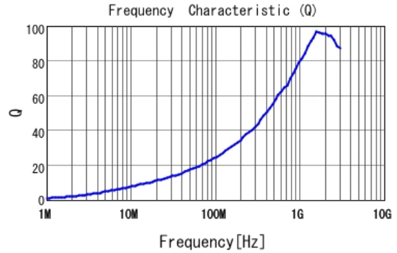
■ LQW15AN9N0G8Z Q
