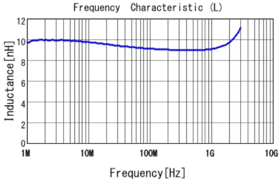
■ LQW15AN9N0G8Z L
