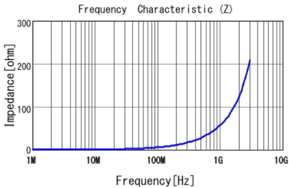
■ LQW15AN9N0G80 |Z|
