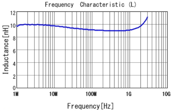
■ LQW15AN9N0G80 L
