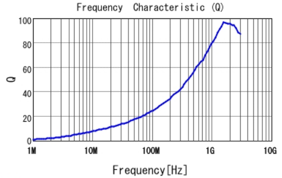
■ LQW15AN9N0G80 Q
