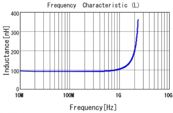
■ LQW15AN91NJ00 L
