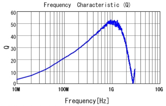
■ LQW15AN91NJ00 Q
