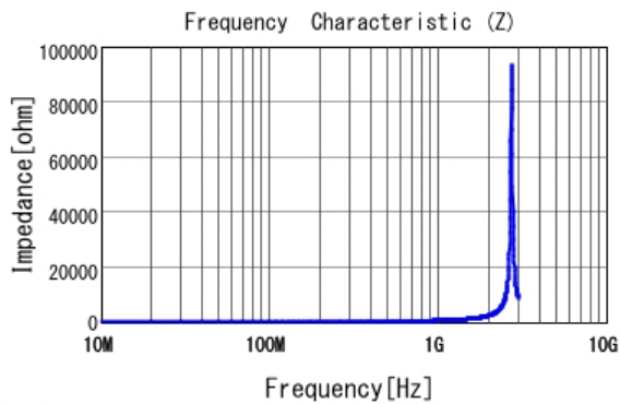
■ LQW15AN91NJ00 |Z|
