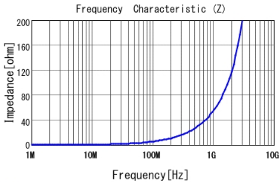
■ LQW15AN8N7G80 |Z|
