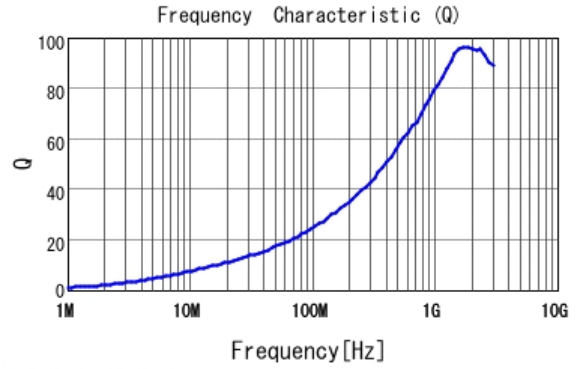
■ LQW15AN8N7G80 Q
