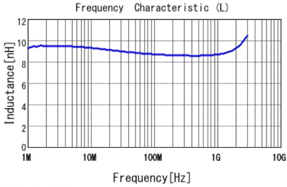
■ LQW15AN8N7G80 L
