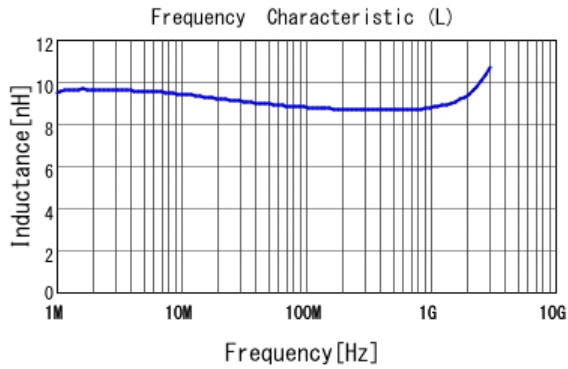
■ LQW15AN8N6G8Z L
