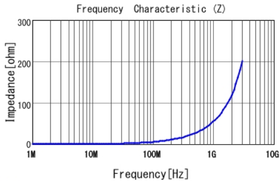
■ LQW15AN8N6G8Z |Z|
