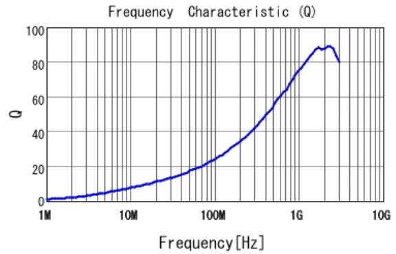
■ LQW15AN8N6G8Z Q
