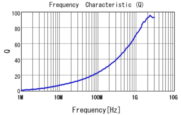
■ LQW15AN8N2J8Z Q
