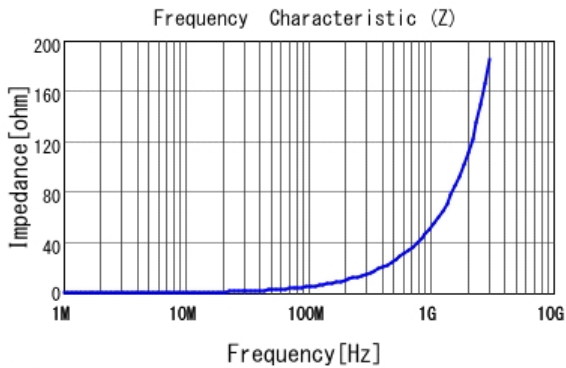
■ LQW15AN8N2J8Z |Z|
