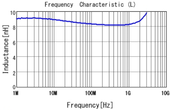
■ LQW15AN8N2J8Z L
