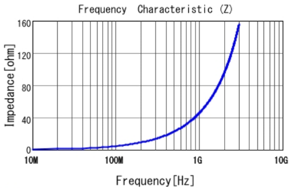
■ LQW15AN7N3H00 |Z|
