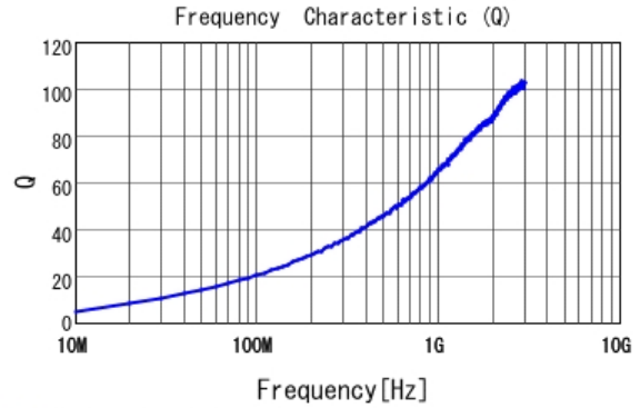
■ LQW15AN7N3H00 Q
