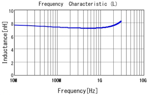
■ LQW15AN7N3H00 L
