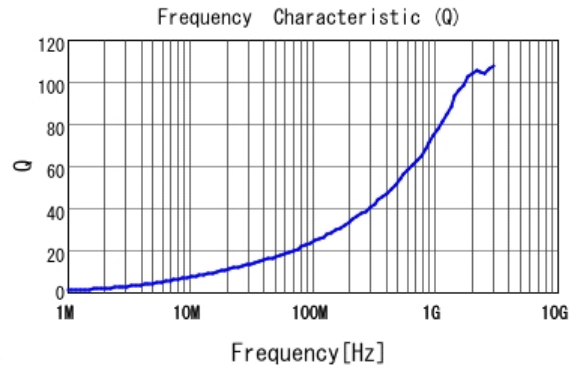
■ LQW15AN7N0G80 Q
