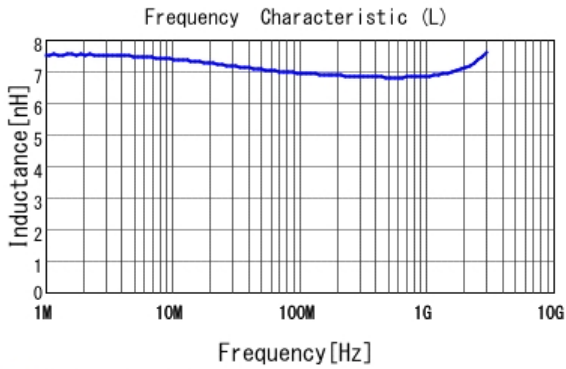
■ LQW15AN7N0G80 L
