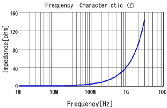
■ LQW15AN7N0G80 |Z|
