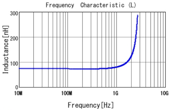
■ LQW15AN72NG00 L
