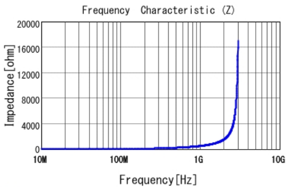
■ LQW15AN72NG00 |Z|
