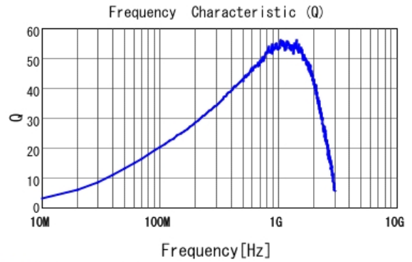
■ LQW15AN72NG00 Q
