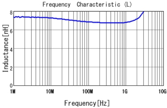
■ LQW15AN6N8G8Z L
