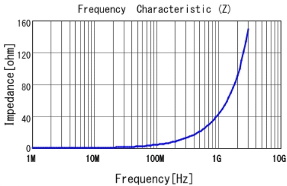
■ LQW15AN6N8G8Z |Z|
