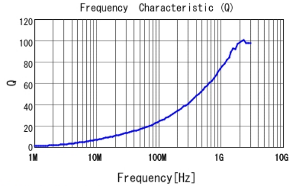
■ LQW15AN6N8G8Z Q
