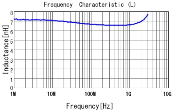
■ LQW15AN6N6G8Z L
