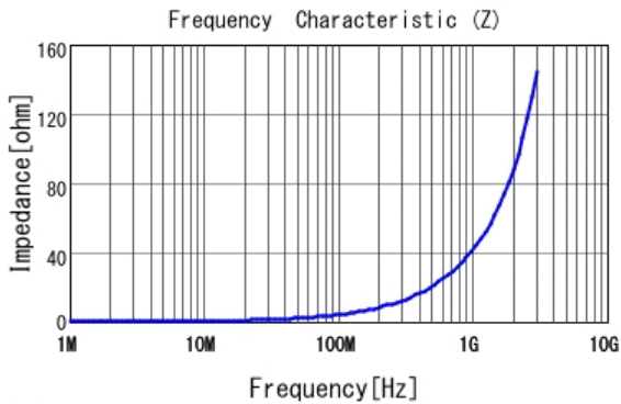
■ LQW15AN6N6G8Z |Z|
