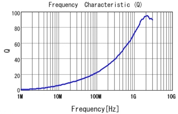
■ LQW15AN6N6G8Z Q
