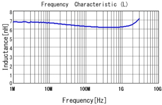
■ LQW15AN6N4G8Z L
