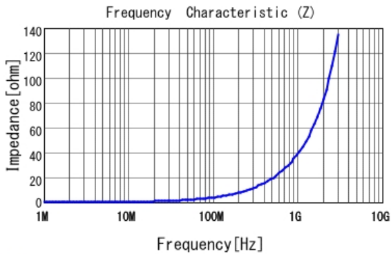
■ LQW15AN6N4G8Z |Z|
