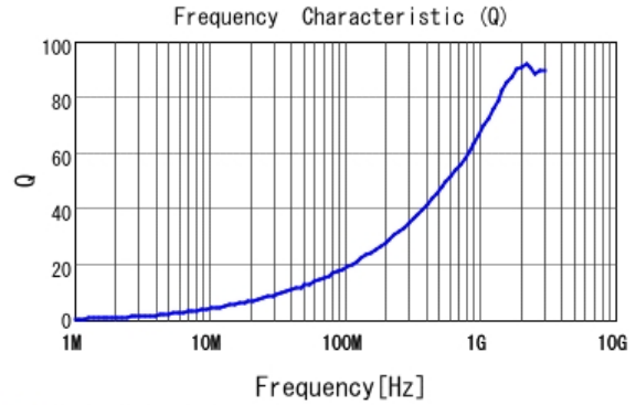
■ LQW15AN6N4G8Z Q
