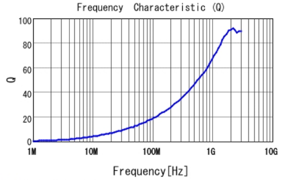
■ LQW15AN6N4G80 Q
