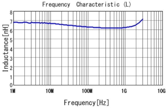
■ LQW15AN6N4G80 L
