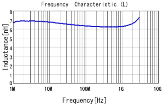
■ LQW15AN6N3G80 L
