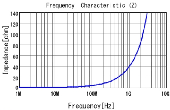
■ LQW15AN6N3G80 |Z|
