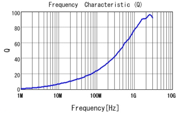
■ LQW15AN6N3G80 Q
