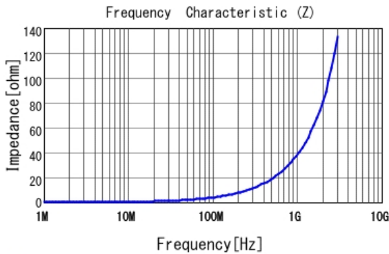
■ LQW15AN6N2G80 |Z|
