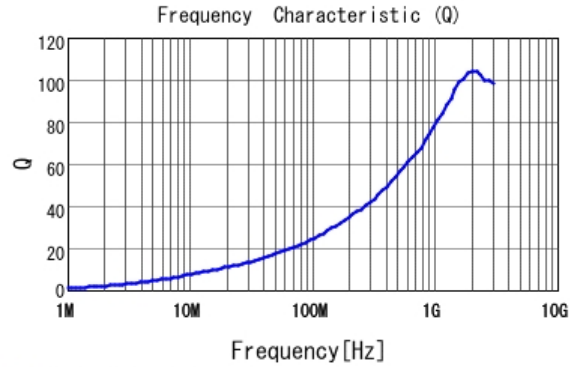
■ LQW15AN6N2G80 Q
