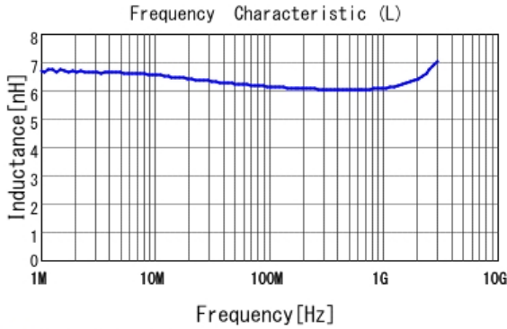
■ LQW15AN6N2G80 L
