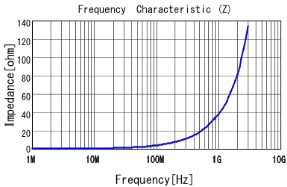
■ LQW15AN6N1D8Z |Z|
