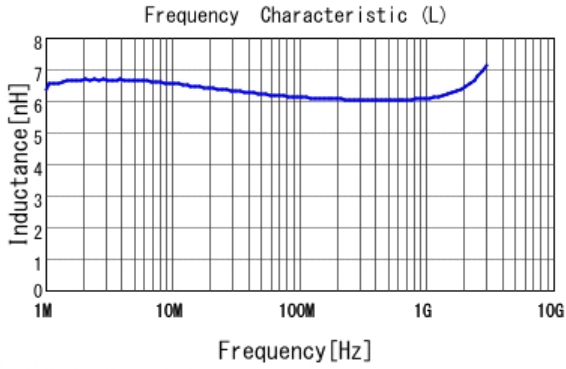
■ LQW15AN6N1D8Z L
