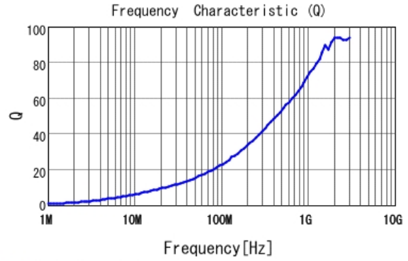
■ LQW15AN6N1D8Z Q
