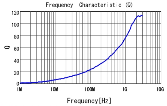
■ LQW15AN6N0B80 Q
