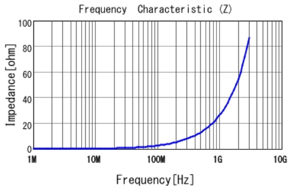
■ LQW15AN6N0B80 |Z|
