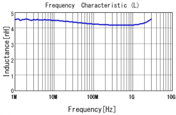
■ LQW15AN6N0B80 L
