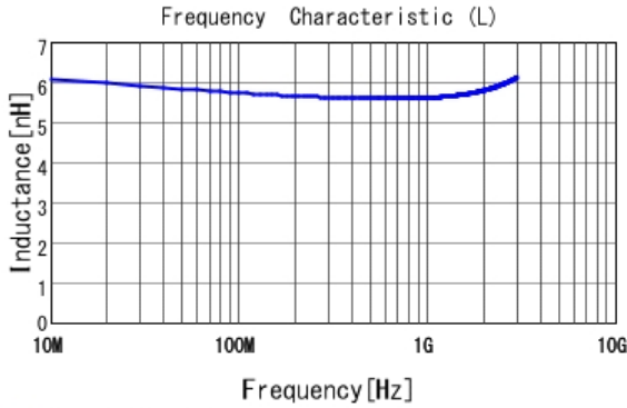
■ LQW15AN5N8D00 L
