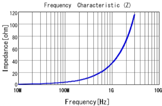
■ LQW15AN5N8D00 |Z|
