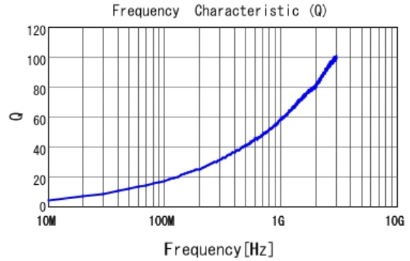
■ LQW15AN5N8D00 Q
