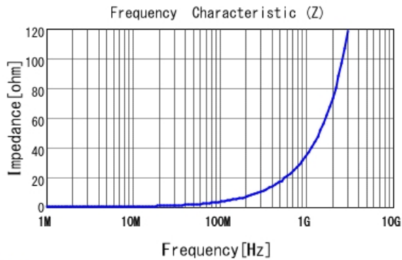
■ LQW15AN5N6G80 |Z|
