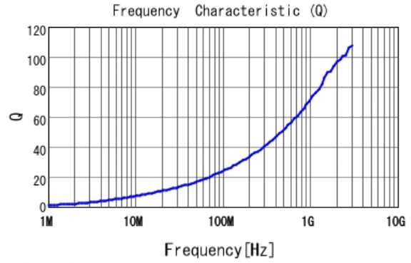
■ LQW15AN5N6G80 Q
