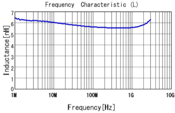
■ LQW15AN5N6G80 L
