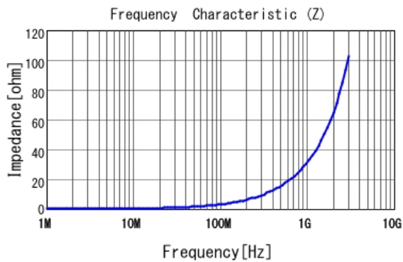
■ LQW15AN5N0D8Z |Z|
