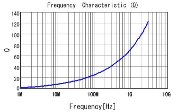
■ LQW15AN5N0D8Z Q
