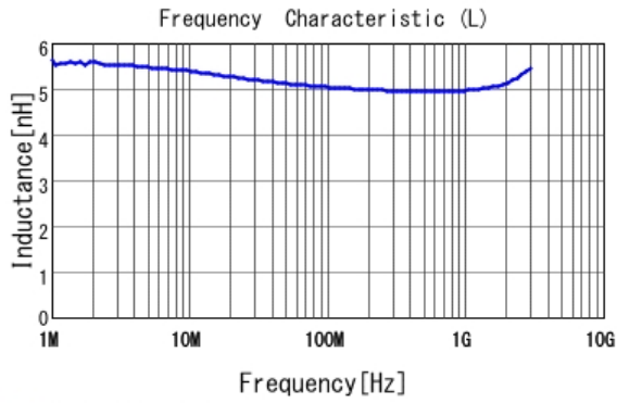
■ LQW15AN5N0D8Z L
