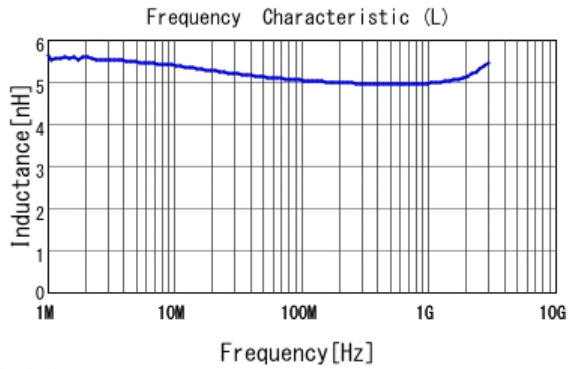
■ LQW15AN5N0B80 L
