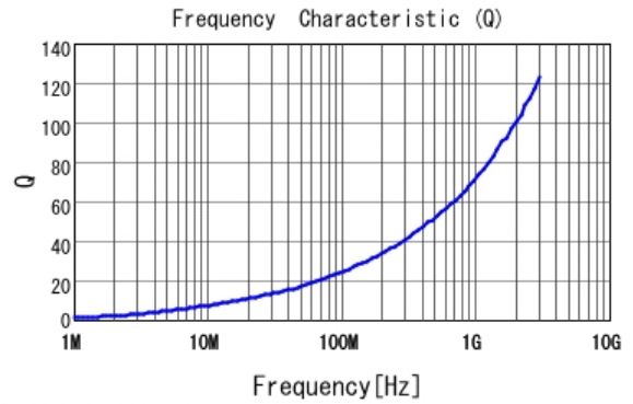
■ LQW15AN5N0B80 Q
