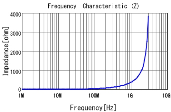
■ LQW15AN56NG8Z |Z|
