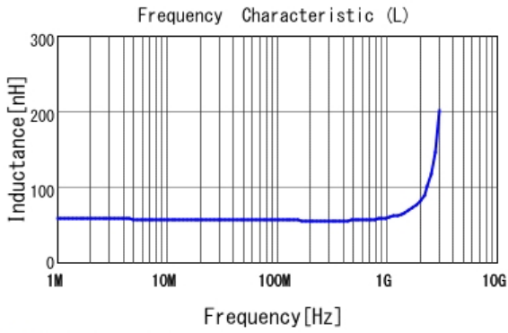
■ LQW15AN56NG8Z L
