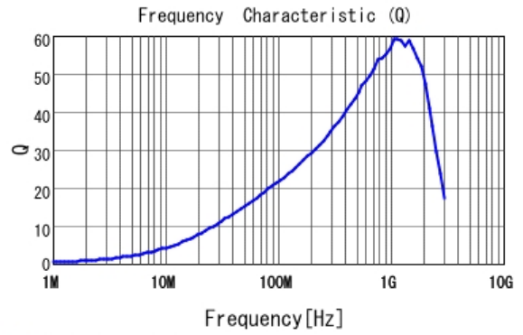
■ LQW15AN56NG8Z Q
