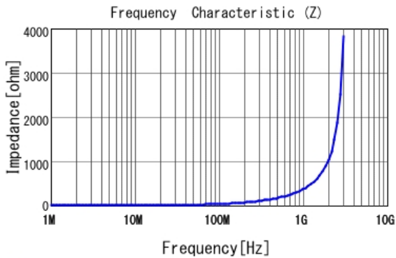
■ LQW15AN56NG80 |Z|
