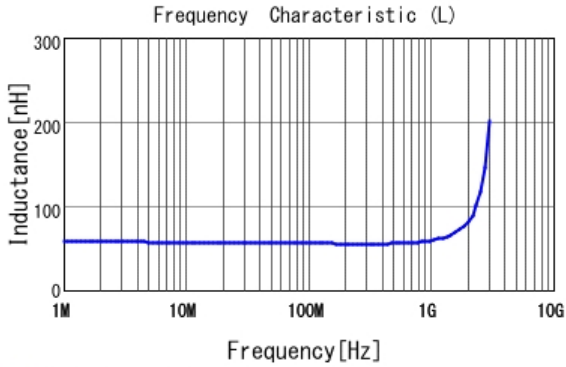
■ LQW15AN56NG80 L
