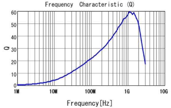
■ LQW15AN56NG80 Q
