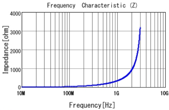
■ LQW15AN51NH00 |Z|
