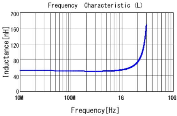
■ LQW15AN51NH00 L
