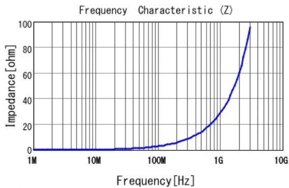
■ LQW15AN4N7G80 |Z|
