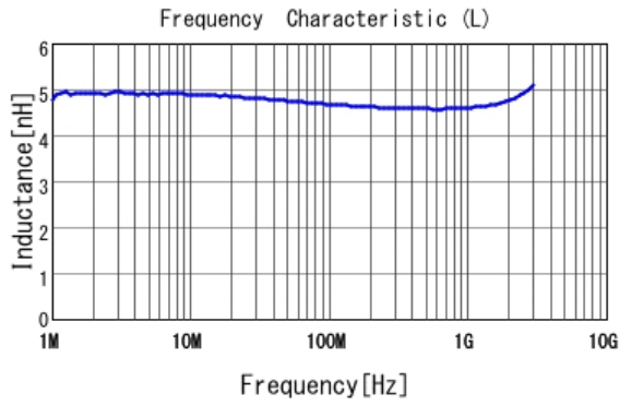
■ LQW15AN4N7G80 L
