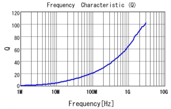
■ LQW15AN4N7G80 Q
