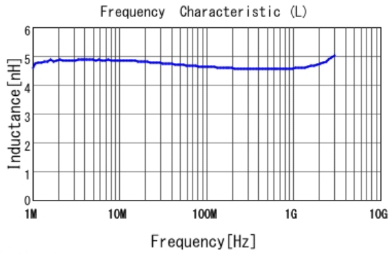
■ LQW15AN4N6G80 L
