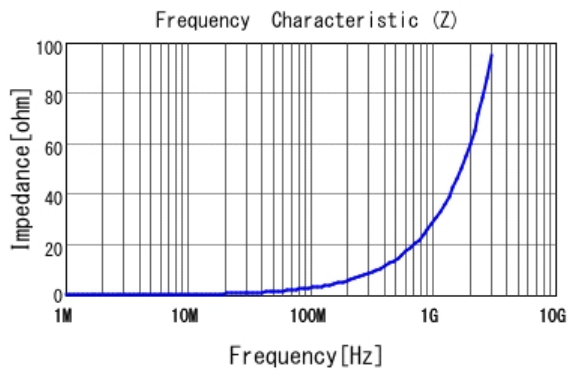
■ LQW15AN4N6G80 |Z|
