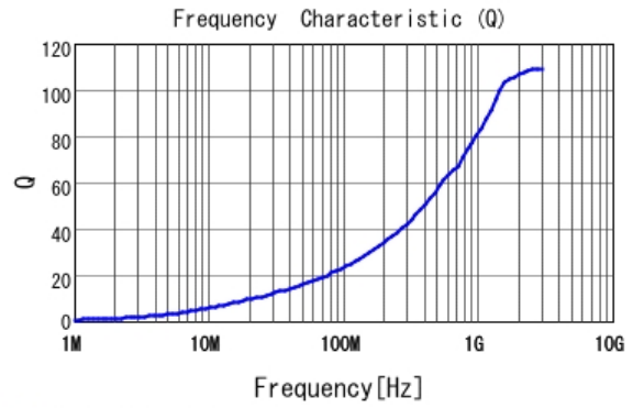
■ LQW15AN4N6G80 Q
