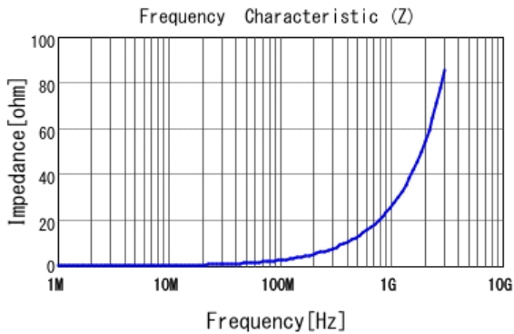
■ LQW15AN4N3G80 |Z|
