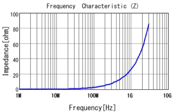
■ LQW15AN4N3B8Z |Z|
