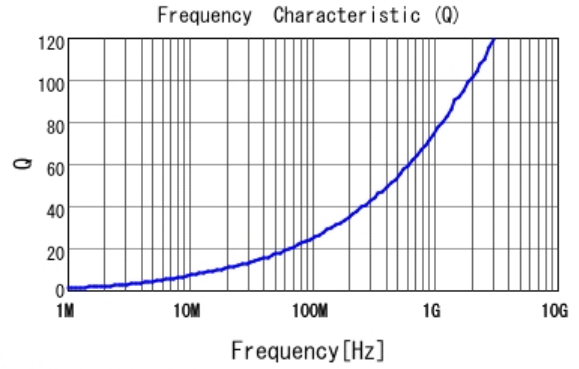
■ LQW15AN4N0G8Z Q
