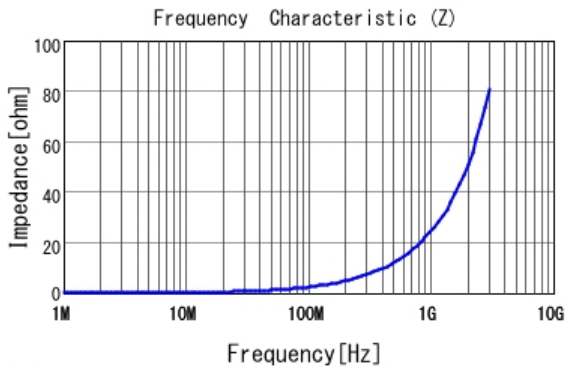
■ LQW15AN4N0G8Z |Z|
