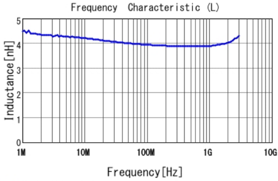
■ LQW15AN4N0G8Z L
