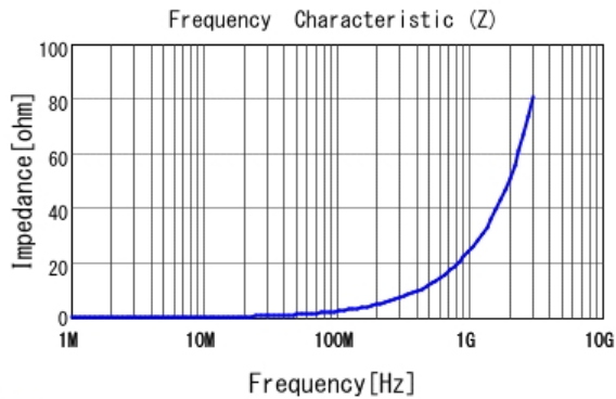
■ LQW15AN4N0G80 |Z|
