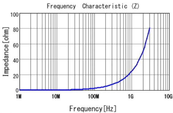
■ LQW15AN4N0B80 |Z|
