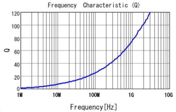
■ LQW15AN4N0B80 Q
