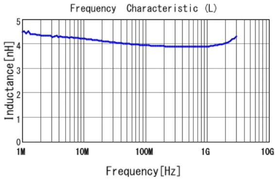
■ LQW15AN4N0B80 L
