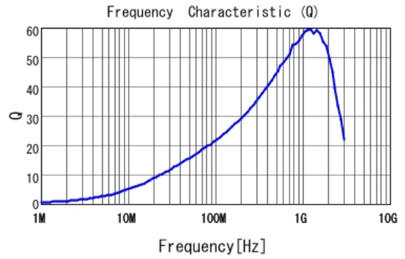
■ LQW15AN47NJ80 Q
