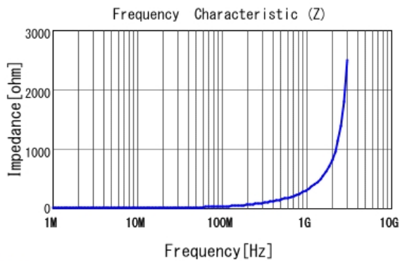
■ LQW15AN47NJ80 |Z|
