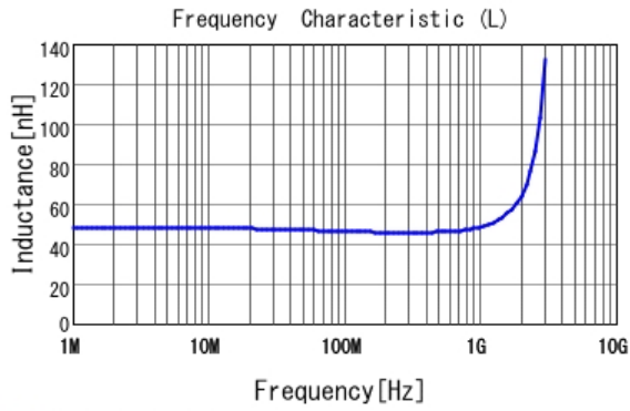
■ LQW15AN47NJ80 L
