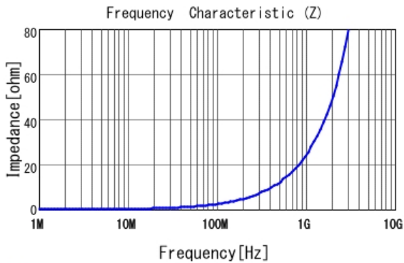
■ LQW15AN3N9G8Z |Z|
