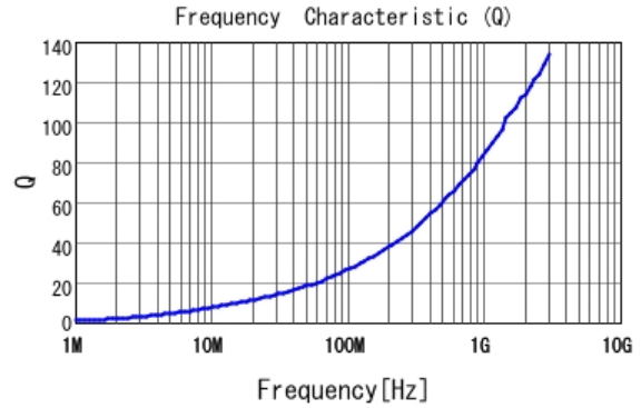
■ LQW15AN3N9G8Z Q
