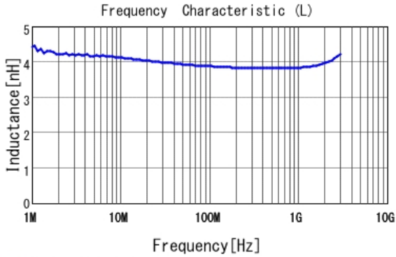
■ LQW15AN3N9G8Z L
