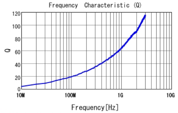
■ LQW15AN3N9B0Z Q
