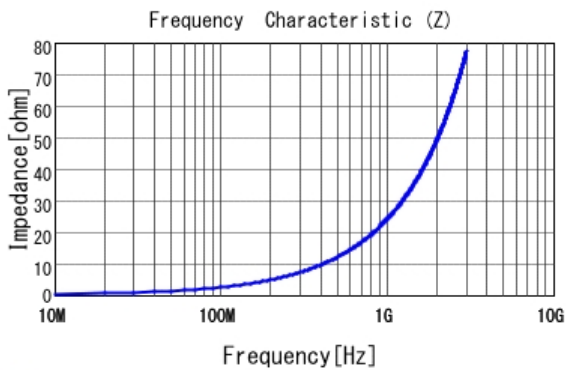
■ LQW15AN3N9B0Z |Z|
