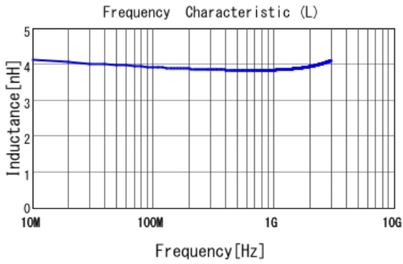
■ LQW15AN3N9B0Z L
