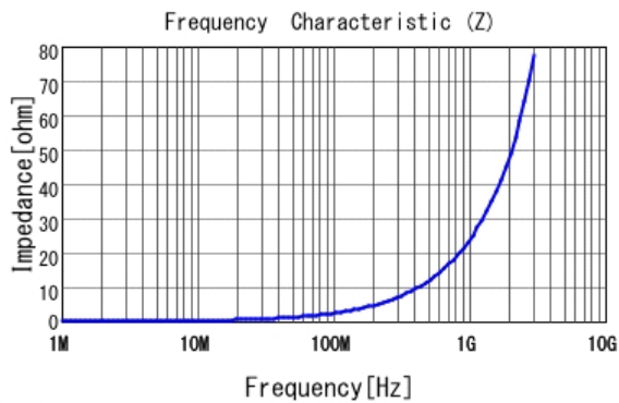
■ LQW15AN3N8G80 |Z|
