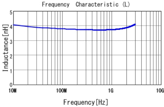
■ LQW15AN3N8C10 L
