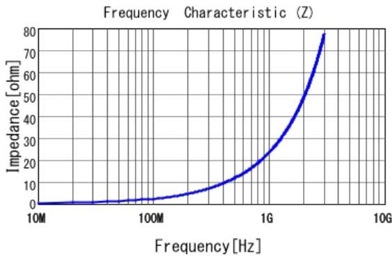
■ LQW15AN3N8C10 |Z|
