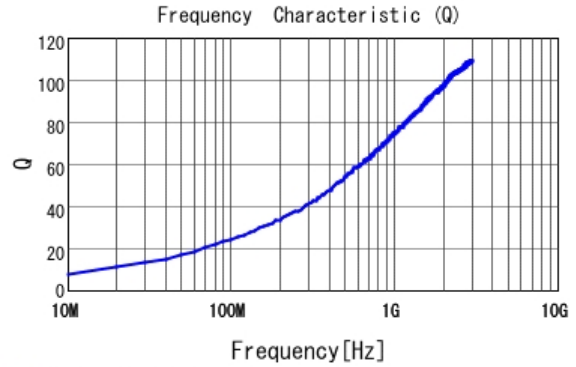
■ LQW15AN3N8C10 Q
