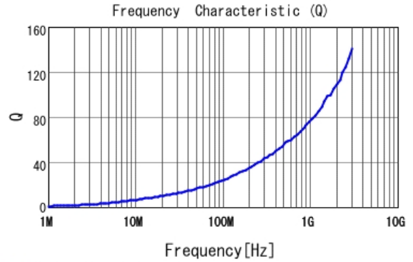
■ LQW15AN3N3G80 Q
