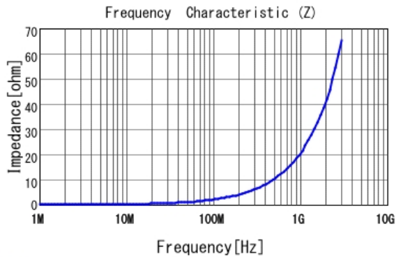
■ LQW15AN3N3G80 |Z|
