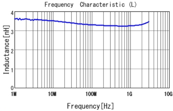
■ LQW15AN3N3G80 L
