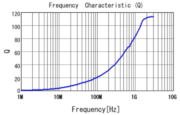
■ LQW15AN3N0G80 Q
