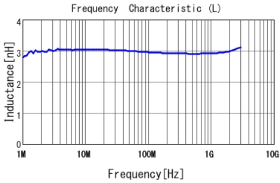
■ LQW15AN3N0G80 L
