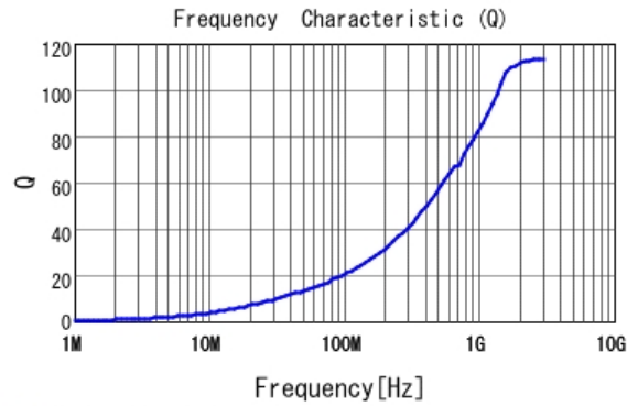
■ LQW15AN3N0B8Z Q
