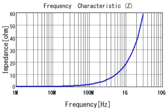
■ LQW15AN3N0B8Z |Z|
