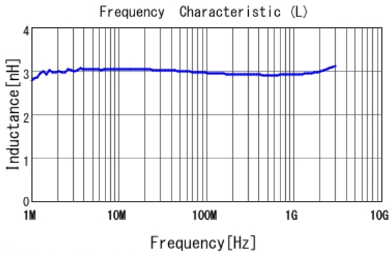
■ LQW15AN3N0B8Z L
