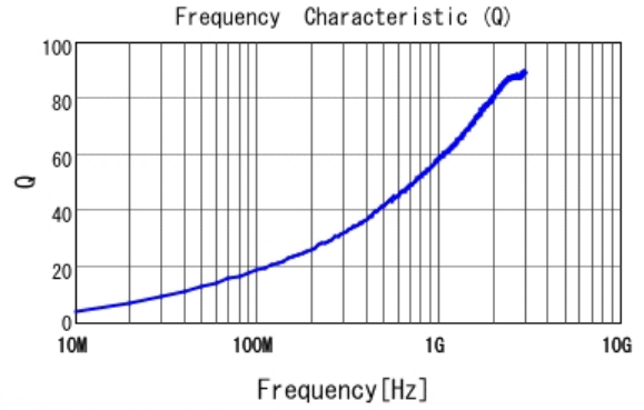
■ LQW15AN3N0B0Z Q
