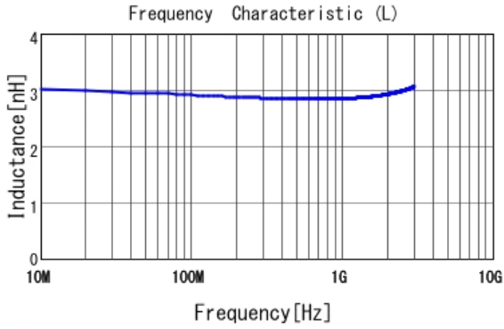
■ LQW15AN3N0B0Z L
