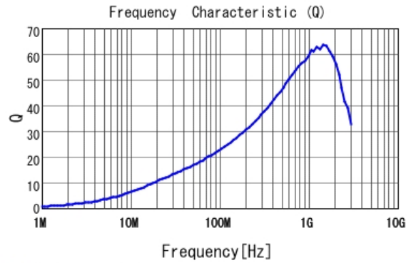
■ LQW15AN39NG8Z Q
