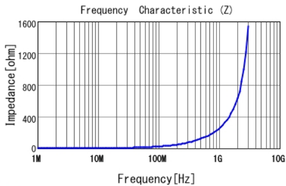
■ LQW15AN39NG8Z |Z|
