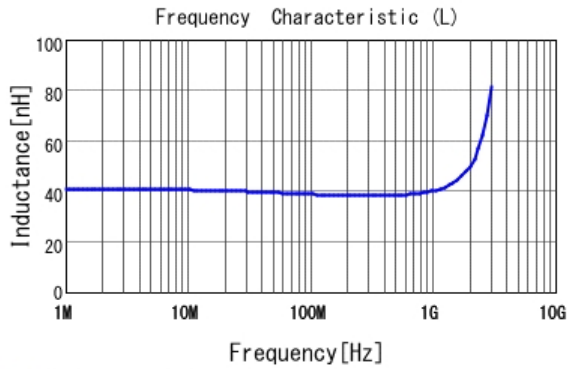
■ LQW15AN39NG8Z L
