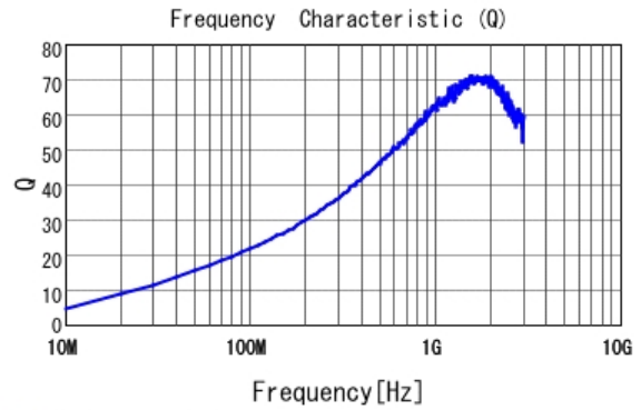
■ LQW15AN39NG0Z Q
