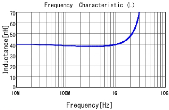
■ LQW15AN39NG0Z L
