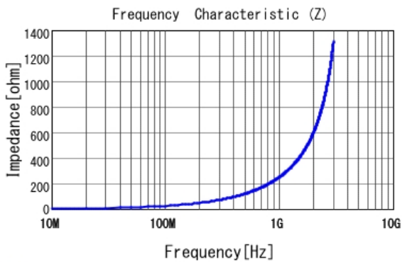
■ LQW15AN39NG0Z |Z|
