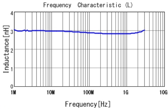
■ LQW15AN2N9G80 L
