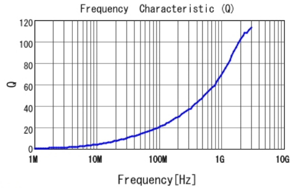
■ LQW15AN2N9G80 Q
