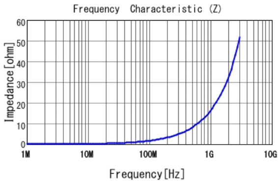
■ LQW15AN2N7G8Z |Z|
