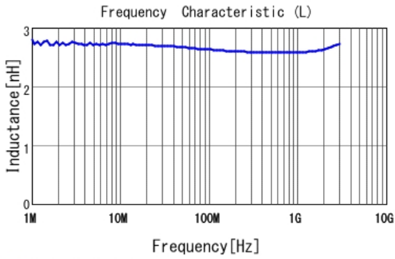
■ LQW15AN2N7G8Z L
