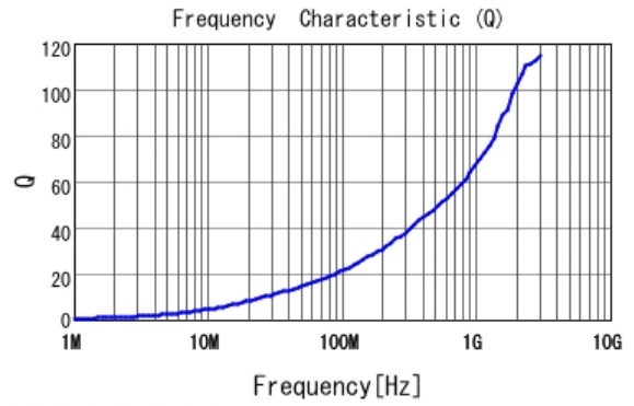
■ LQW15AN2N7G8Z Q
