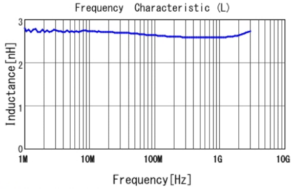
■ LQW15AN2N7G80 L
