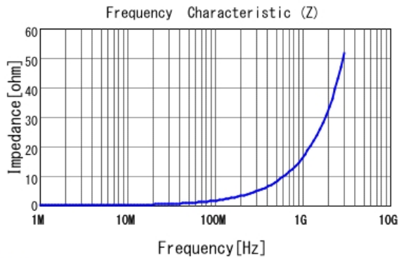
■ LQW15AN2N7G80 |Z|
