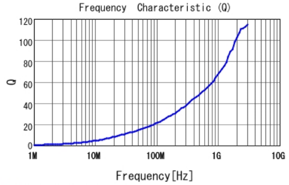
■ LQW15AN2N7G80 Q
