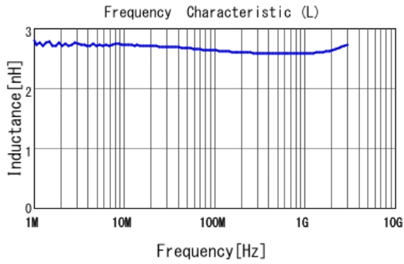
■ LQW15AN2N7B8Z L
