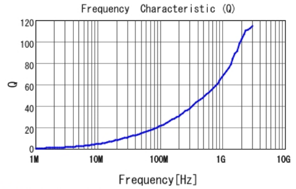
■ LQW15AN2N7B8Z Q
