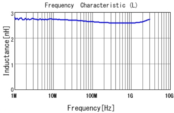
■ LQW15AN2N7B80 L
