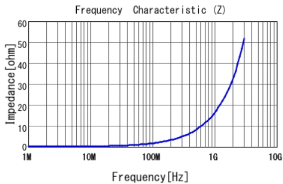
■ LQW15AN2N7B80 |Z|
