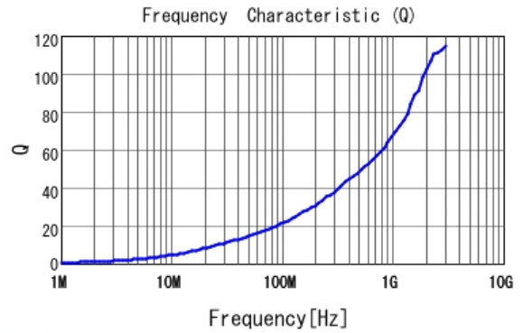
■ LQW15AN2N7B80 Q
