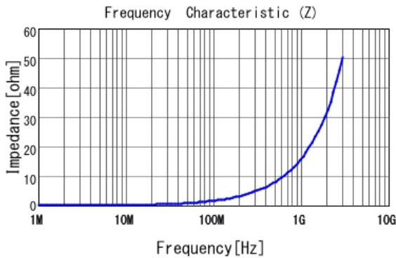
■ LQW15AN2N6B8Z |Z|
