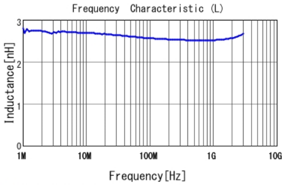
■ LQW15AN2N6B8Z L
