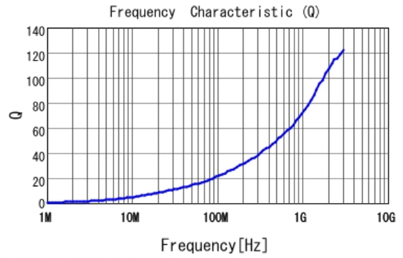
■ LQW15AN2N6B8Z Q
