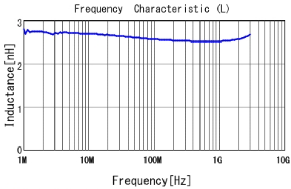
■ LQW15AN2N6B80 L
