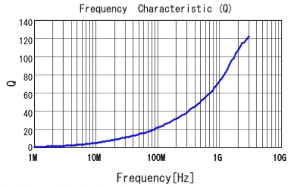
■ LQW15AN2N6B80 Q
