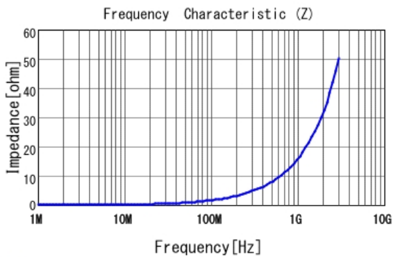
■ LQW15AN2N6B80 |Z|
