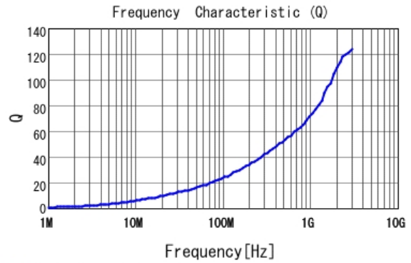
■ LQW15AN2N5G80 Q
